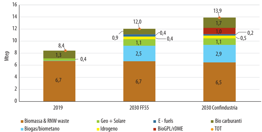
Figura 3.8 Consumi finali di energia da rinnovabili, confronto tra scenario Confindustria, FF55 e dato storico 2019
