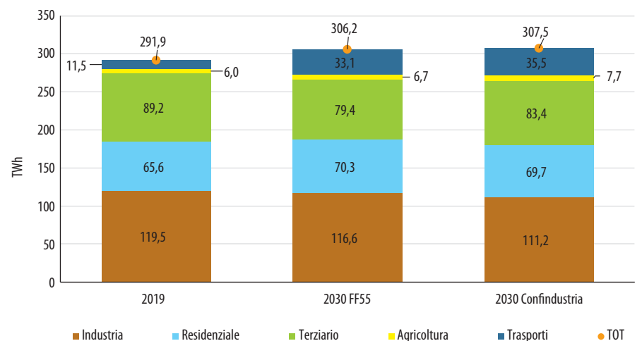
Figura 3.6 Consumi finali elettrici: scenario Confindustria, confronto con lo scenario FF55 e dati storici 2019
