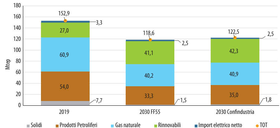
Figura 3.5 Consumi primari di energia, confronto tra scenario Confindustria, FF55 e dato storico 2019
